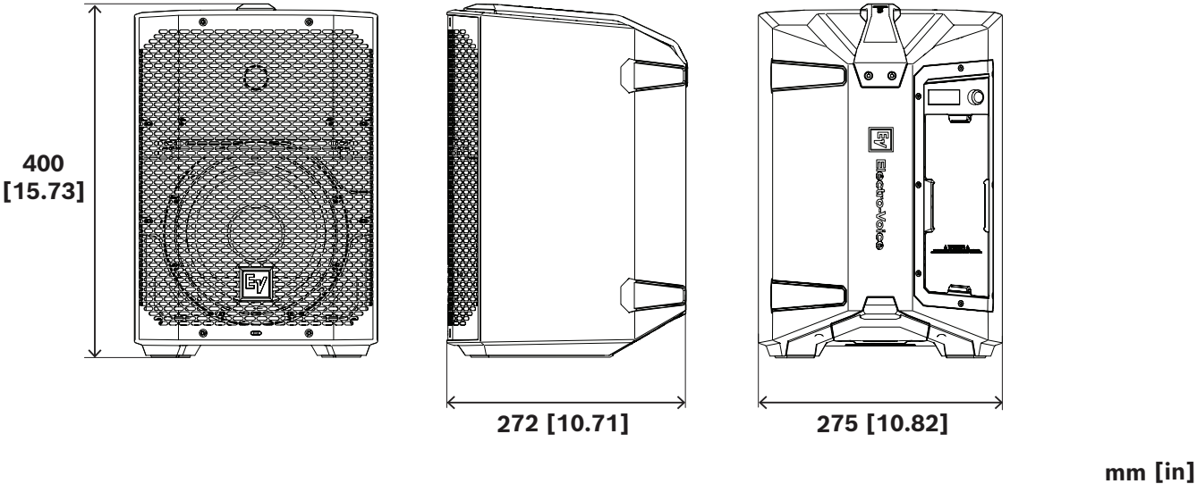
Fig. 1: Dimensions
