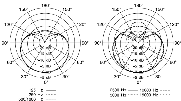
FIGURA 5. DIAGRAMMI POLARI TIPICI
