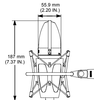
ABBILDUNG 6. ABMESSUNGEN
