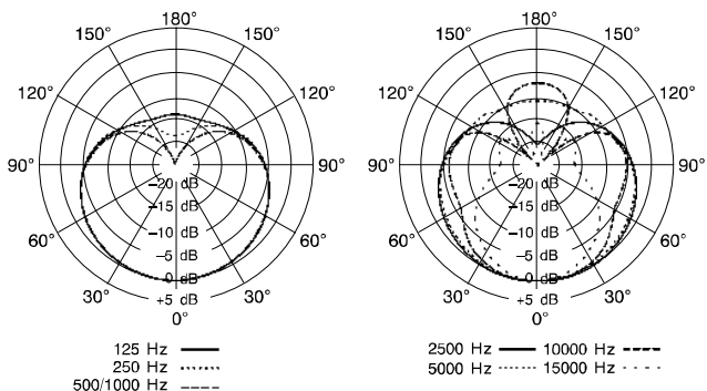
ABBILDUNG 5. TYPISCHE RICHTCHARAKTERISTIK
