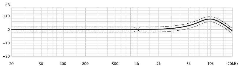
KM 183
