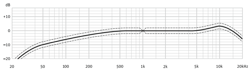
KM 185
