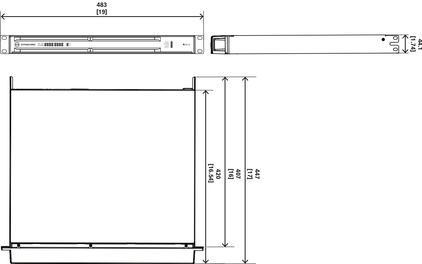
Fig. 3: Dante Router
