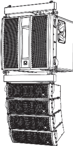
Exemple montrant un ensemble mixte avec 1 subwoofer TLX212L, 4 enceintes TLX43 et 2 flybars TLX43-FLB.
