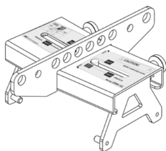
Fly Bar DRK-IG
