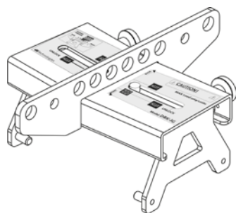
Fly Bar DRK-IG
